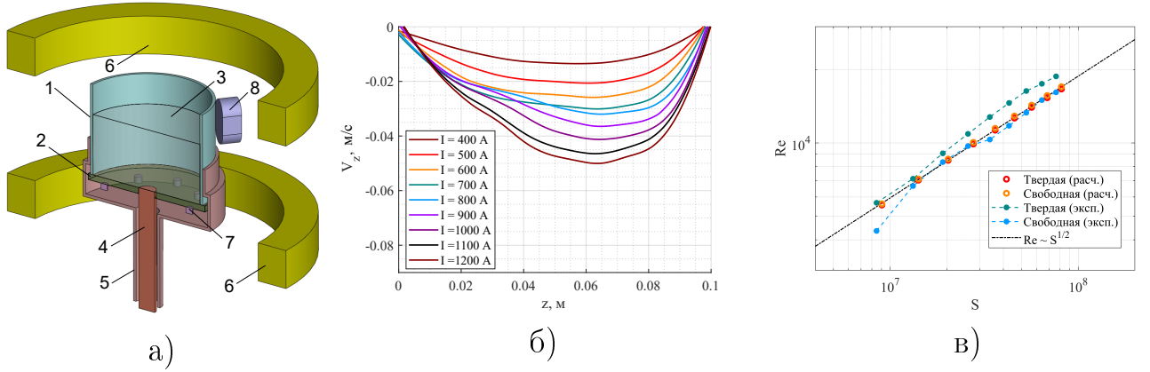
Рис. 4. (а) – схема экспериментальной установки для изучения ЭВТ со свободной поверхностью: 1 – боковая стенка цилиндрической ячейки из нержавеющей стали; 2 – дно ячейки из органического стекла; 3 – жидкий металл; 4 – центральный медный электрод (катод); 5 – внешний медный электрод (анод); 6 – катушки Гельмгольца; 7 – датчики ультразвукового доплеровского анемометра; 8 – индукционный датчик уровня; (б) – профили средней вертикальной скорости V_z , усредненные по датчикам УДА, при различных значениях электрического тока I ; (в) – число Рейнольдса Re в зависимости от ЭВТ-параметра S . Для сплошной верхней границы экспериментальные данные показаны зелеными точками, расчетные данные – красные кружки; для свободной поверхности синие точки – эксперимент, желтые кружки – расчет.
